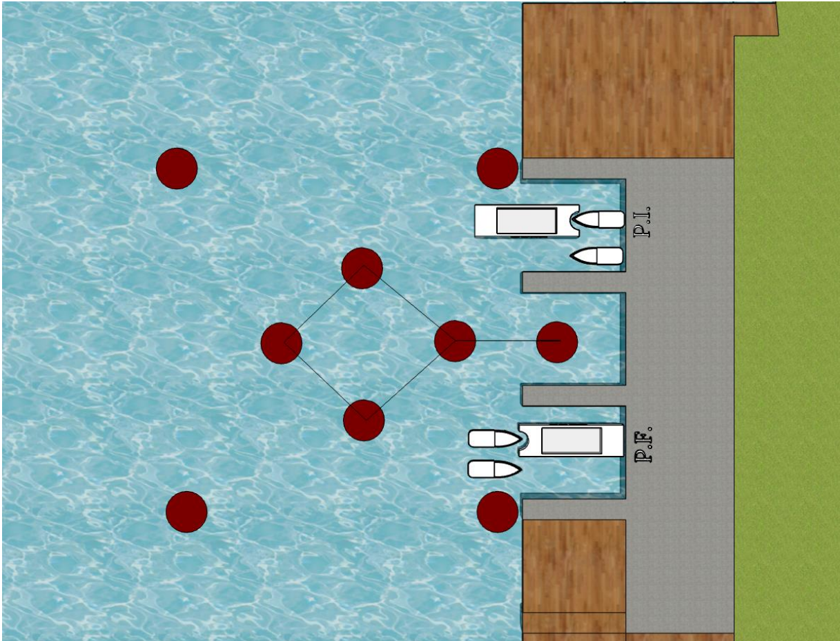
Figura 6 – Desenho esquemático da vista superior do posicionamento das boias.
