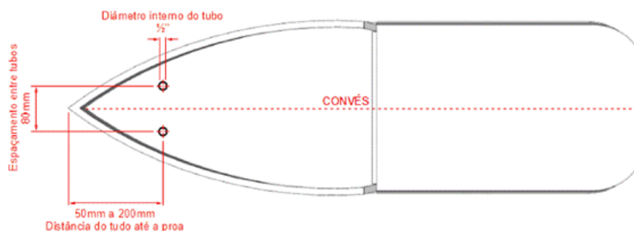
Figura 10 – Ilustração da posição dos tubos de fixação
