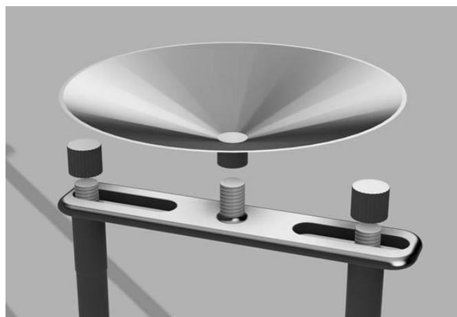
Figura 12 – Detalhe da braçadeira e dos parafusos de encaixe do prato nos tubos de fixação
